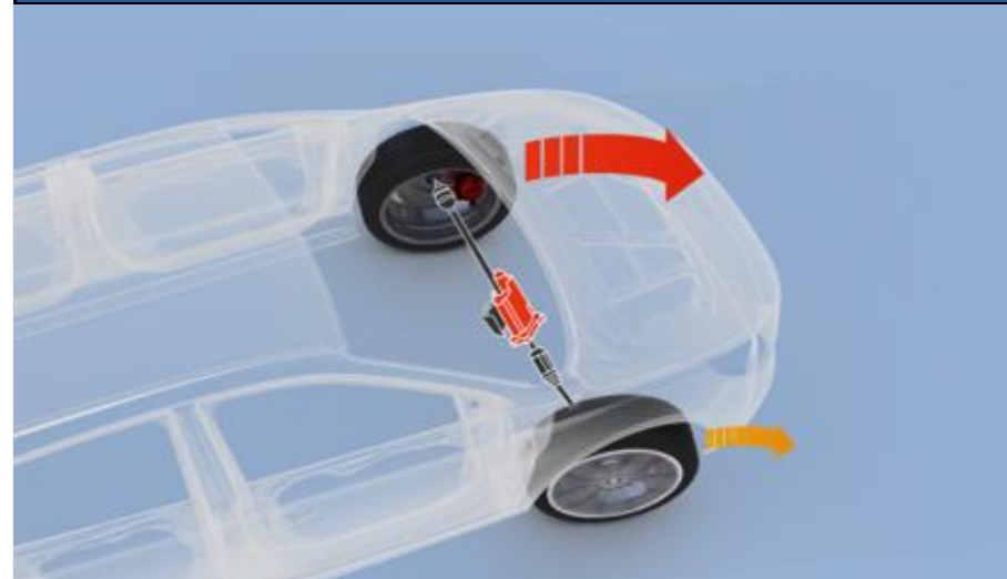
Mechaninis riboto slydimo diferencialas (m-LSD)
